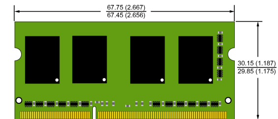
SO-DIMM JEDEC MO-268 204 PIN
