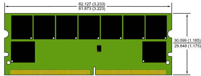
MINI-UDIMM JEDEC MO-244 244 PIN
