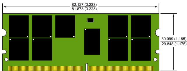
MINI-RDIMM JEDEC MO-244 244 PIN
