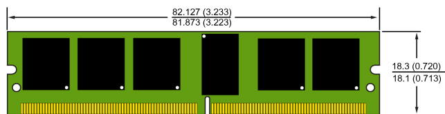
MINI-RDIMM VLP JEDEC MO-244 244 PIN
