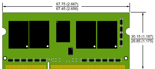
SO-RDIMM JEDEC MO-268 204 PIN
