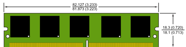
MINI-UDIMM VLP JEDEC MO-244 244 PIN
