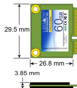
mSATA MINI SATA III
